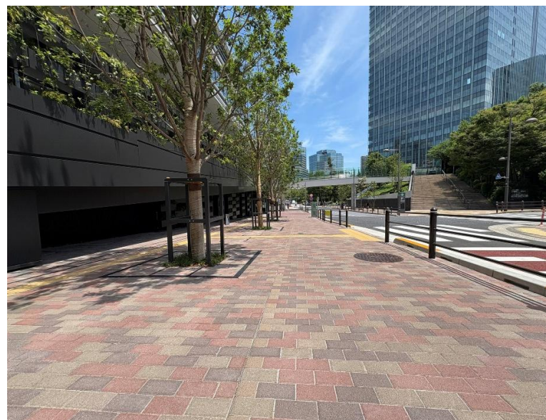
保水ブロック：大崎駅西口（東京都品川区）
