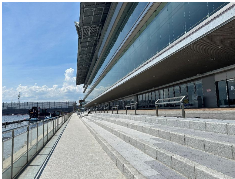
遮熱ブロック：ポートレース津（三重県津市）
